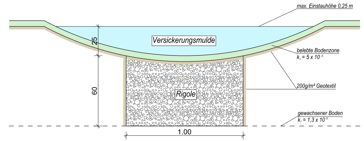
Schemaschnitt Mulden-Rigolen-Element
